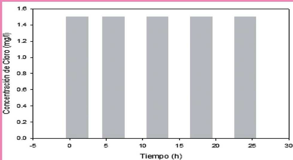
Figura 2. Concentración de cloro obtenido dentro de la red después de la simulación (EPANET) con la activación de tanques elevados y cloradores.
