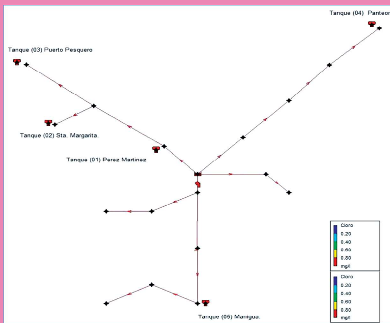
Figura 1. Diagrama de EPANET
